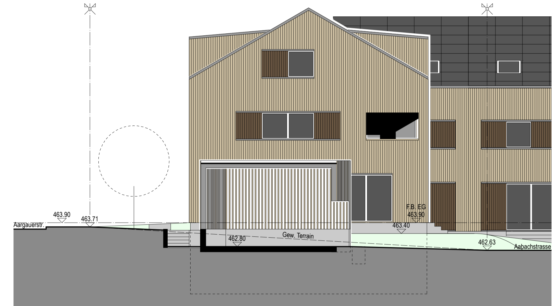
Schnitt / Ansicht B-B
